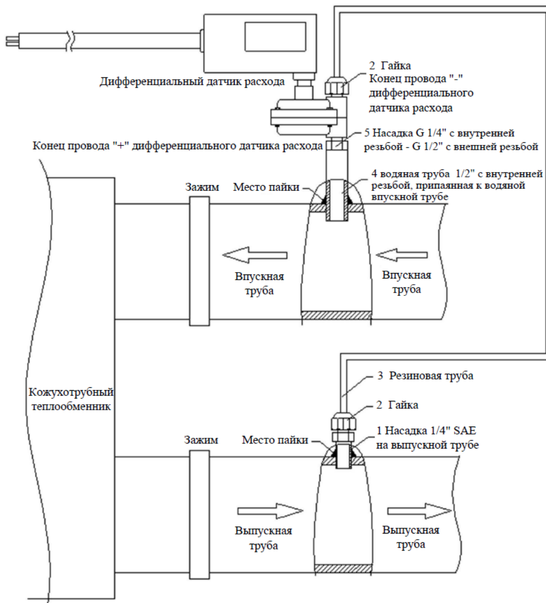
Рис. 5. Схема установки дифференциального реле расхода кожухотрубного теплообменника
